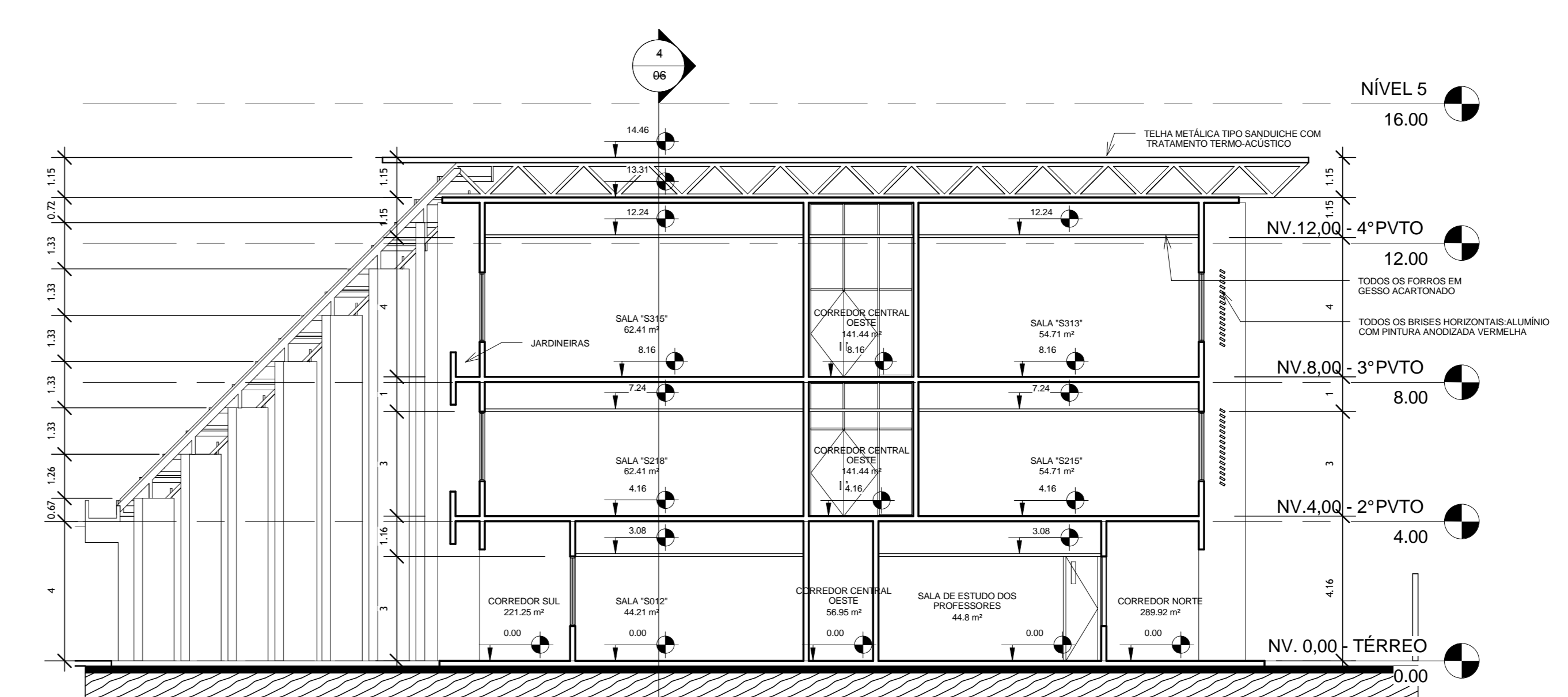
CORTE 11 - SALAS AULA S
